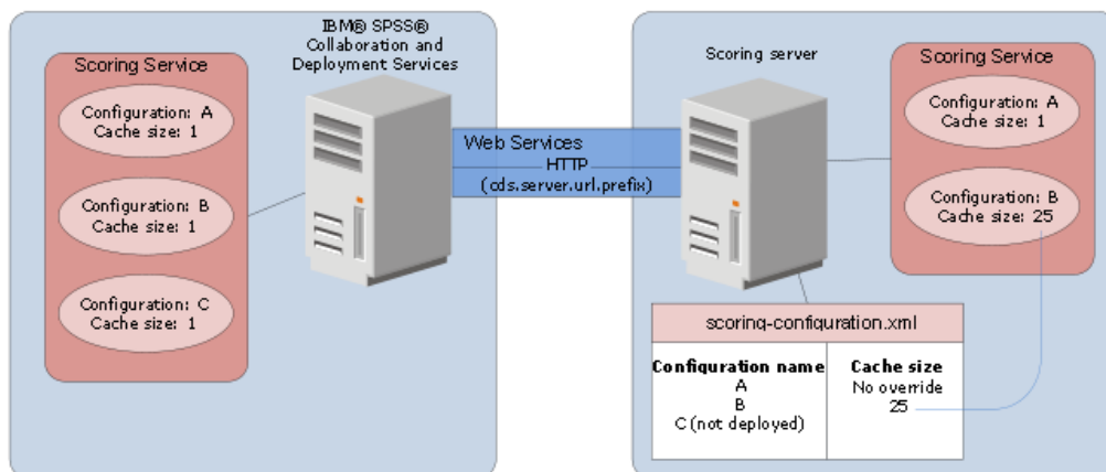
Figura 4. Configuración de entorno de servidor de puntuación
